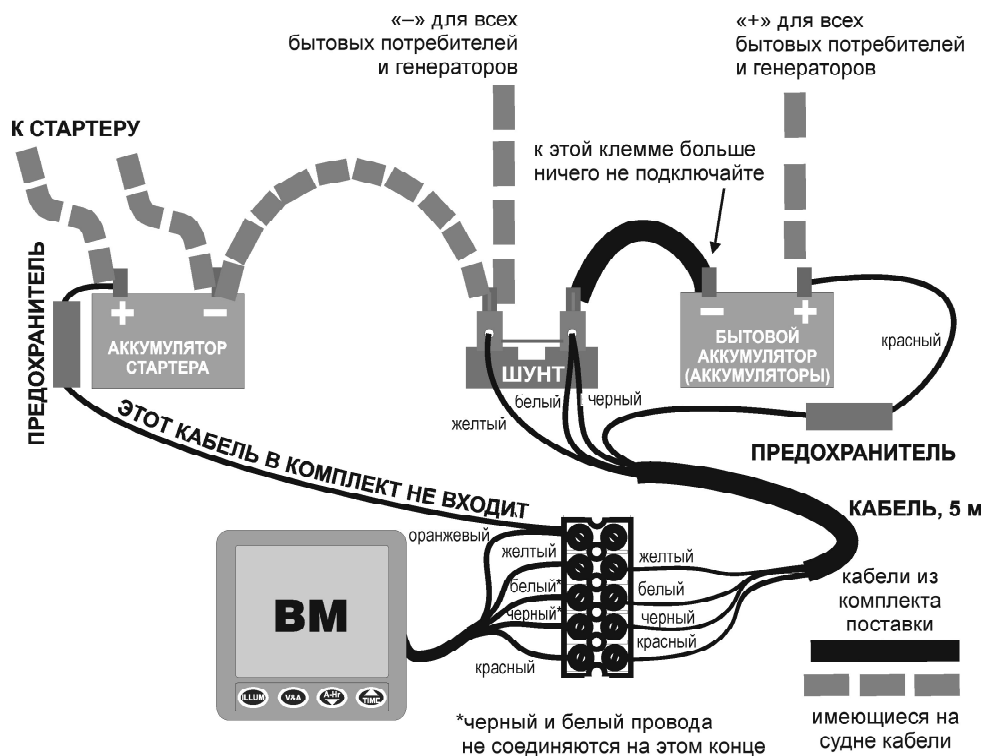
Рис. 2. Схема подключения прибора к бытовому аккумулятору (аккумуляторам) и аккумулятору стартера
